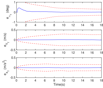
(d) EKF target state errors: Pursuer 2
