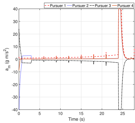
(d) Pursuer control inputs
