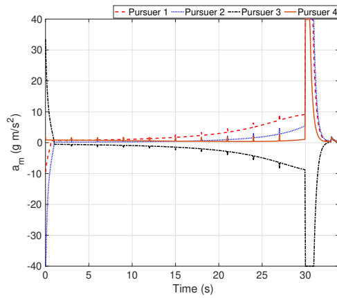
(d) Pursuer control inputs
