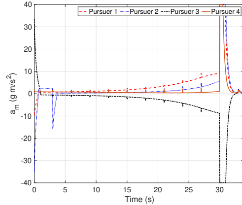
(d) Pursuer control inputs
